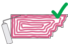
PU penu naneti kružno pomoću aplikatora na fasadni profil po celoj površini koja se lepi, kako bi se sprečio prodor vode iza profila
